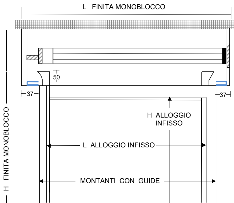
Montanti con guide
