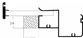
Traverso con blocca cielino
