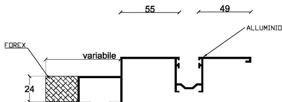
Montanti con guide
