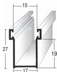
Cod. TS 1727/... 17 x 27 mm
