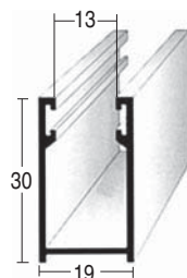
Cod. TS 1930/... 19 x 30 mm
