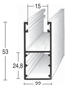
Cod. TS 2253/... 22 x 53 mm
