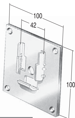
SUPPORTO ZINCATO PER FIANCO TS 300F 45
