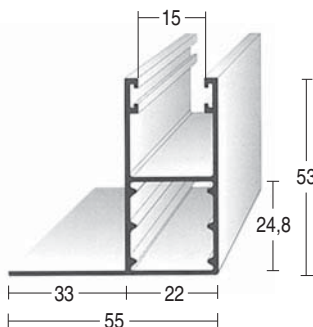
Cod. TS 2253 33/... 22 x 53 mm
