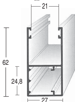
Cod. TS 2762/... 27 x 62 mm
