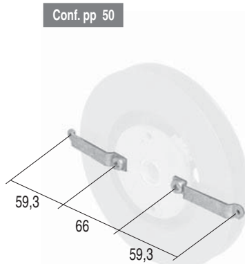
STAFFE DI FISSAGGIO IN ACCIAIO PER MINI RIDUTTORE
