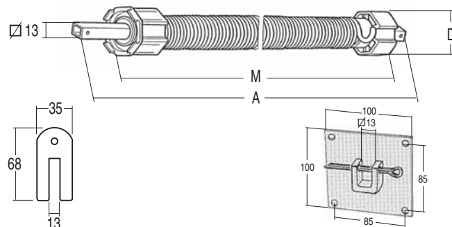
MOLLA DI COMPENSAZIONE CON CAVALLOTTO DI ARRESTO E SUPPORTO
