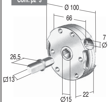
ARGANELLO K 30 AD ASTA RAPP. 1 : 11 CON FINE CORSA - INNESTO Ø 15
