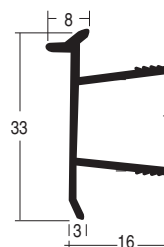
Cod. TS 0935/... 33 x 16 mm
