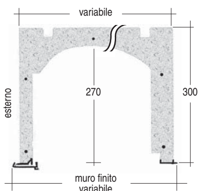
TS BLOCK R ristretto
