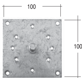
SUPPORTO ZINCATO PERNO Ø 12 PER ARGANELLI K30
