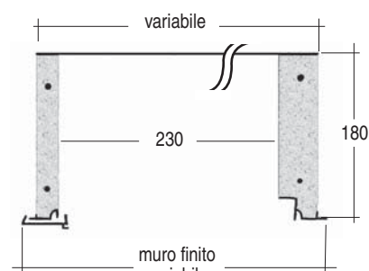
TS BLOCK RIB ribassato
